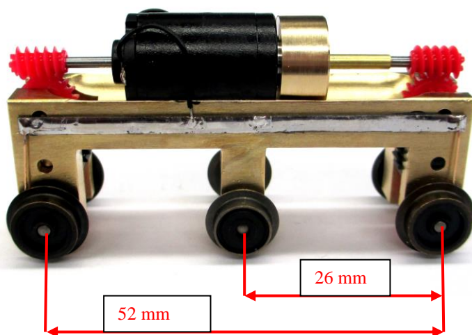
Straßenbahntriebwagen Typ T23 der Bahnen der Stadt Köln, Baugröße H0
