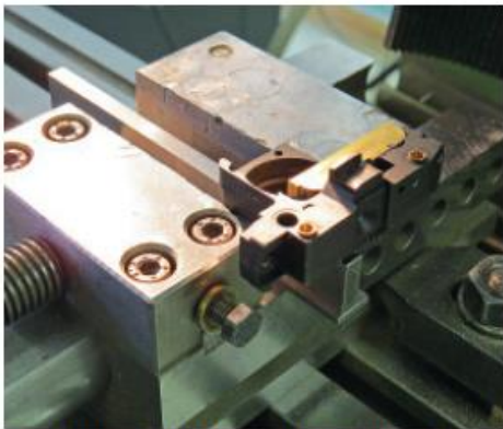
Der Original Trix-Motorhalter besteht aus Druckguss. Dieser ist leider...
